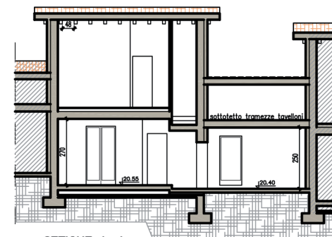
SEZIONE A-A
