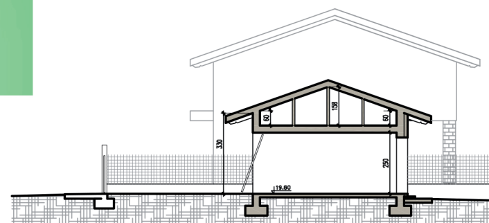
SEZIONE D-D
