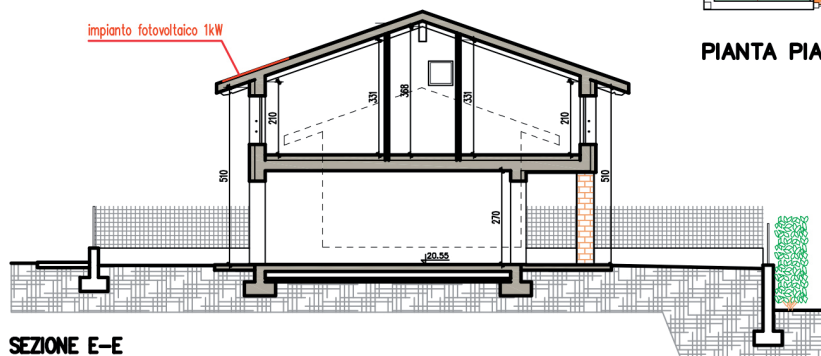
SEZIONE E-E
