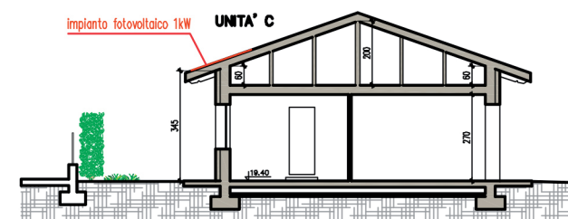
SEZIONE C-C
