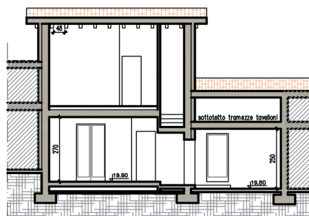
SEZIONE A-A
